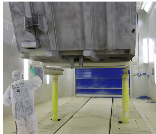
Manuelle Beschichtung von Kippern in SLF-Lackierkabine mit integrierter Schwerlast-Hubvorrichtung
